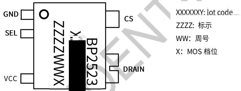
图 2 管脚封装图
