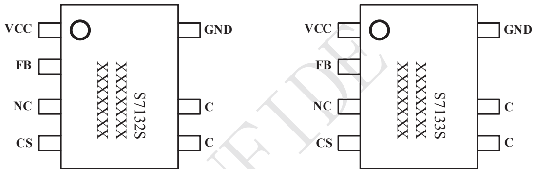
封装管脚图
